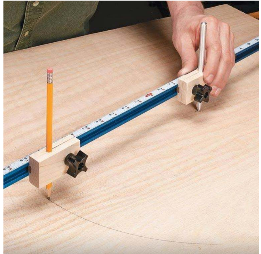
Рейсмус циркуль столярный и строительный
