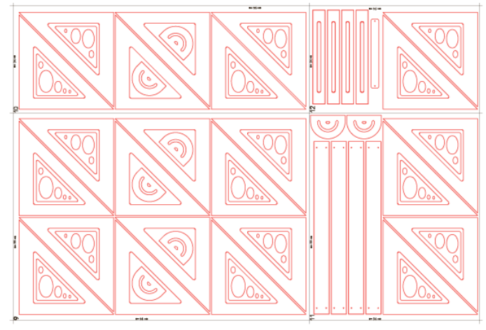
Модель листа для фрезеровки
